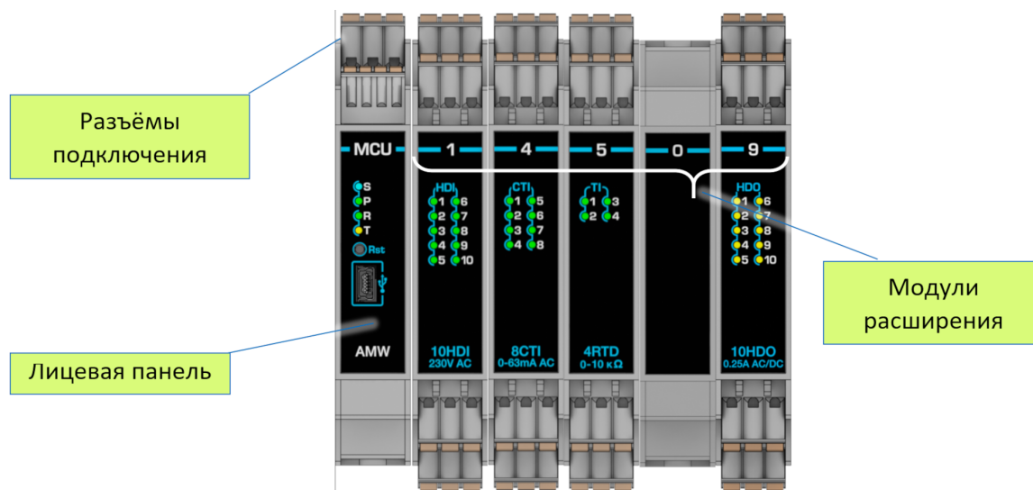
Рисунок 1.2 – Внешний вид устройства
