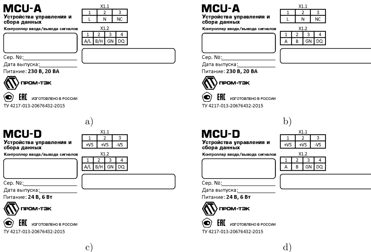
Рисунок 1.5 – Информационная табличка устройств а) MCU-AMW, б) MCU-ARW, в) MCU-DMW, г) MCU-DRW
