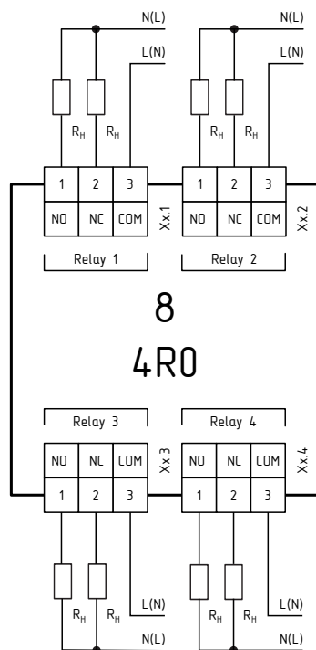
Рисунок 1.22 – Схема подключения модуля расширения MCU-8-4RO
