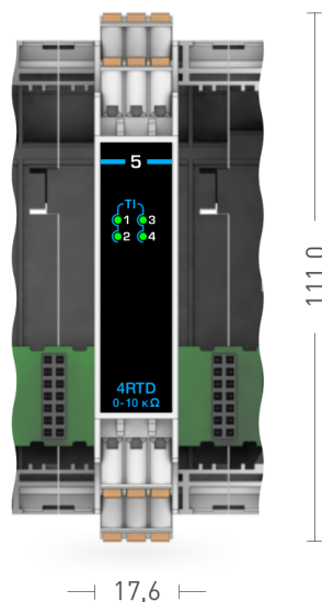
Рисунок 1.15 – Внешний вид модуля расширения MCU-5-4RTD
