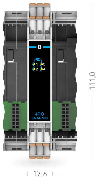
Рисунок 1.21 – Внешний вид модуля расширения MCU-8-4RO
