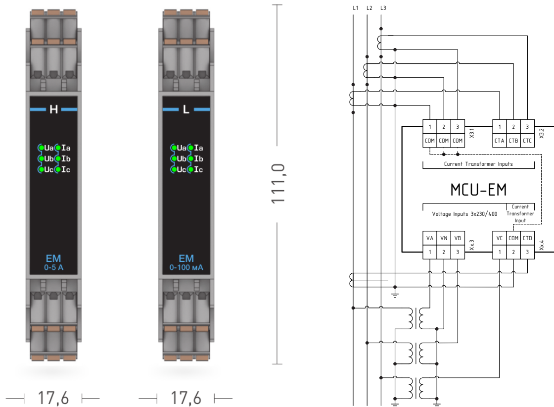
Рисунок 1.25 – Внешний вид и схема подключения модуля расширения EM
