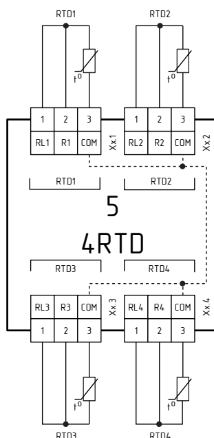
Рисунок 1.16 – Схема подключения модуля расширения MCU-5-4RTD
