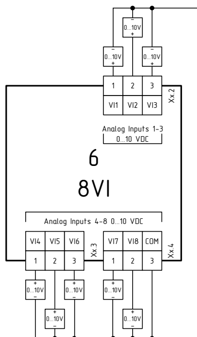
Рисунок 1.18 – Схема подключения модуля расширения MCU-6-8VI
