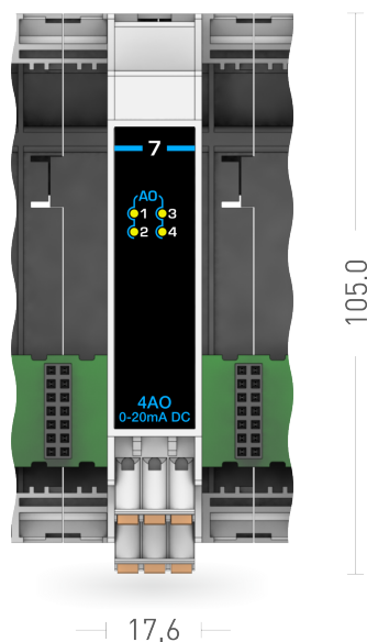
Рисунок 1.19 – Внешний вид модуля расширения MCU-7-4AO
