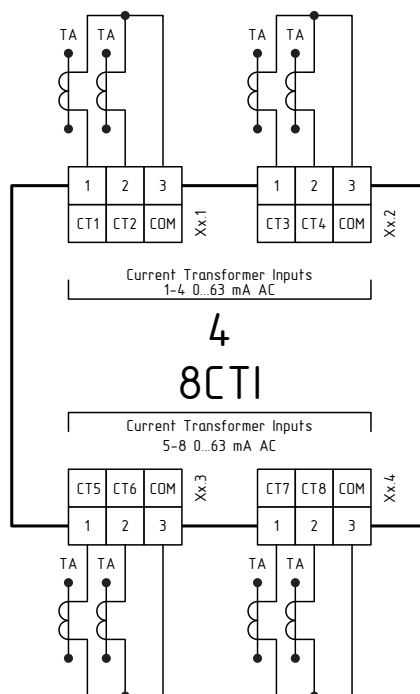
Рисунок 1.14 – Схема подключения модуля расширения MCU-4-8CTI
