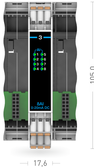
Рисунок 1.11 – Внешний вид модуля расширения MCU-3-8AI
