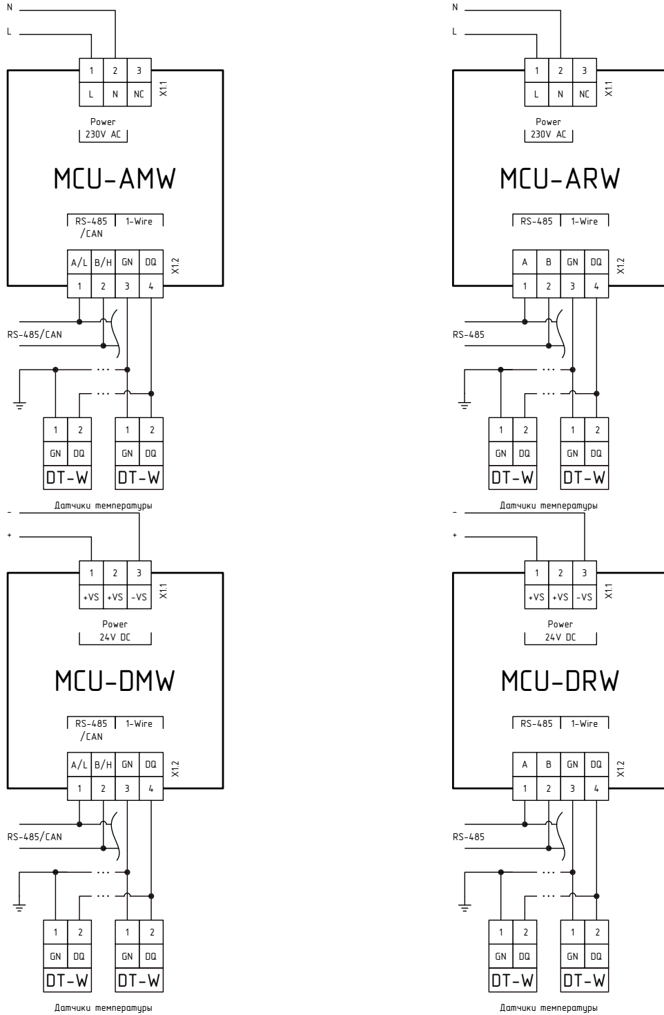
Рисунок 1.6 – Схемы подключения
