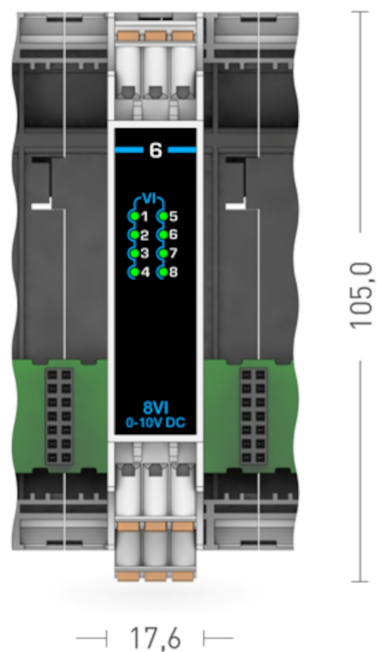
Рисунок 1.17 – Внешний вид модуля расширения MCU-6-8VI
