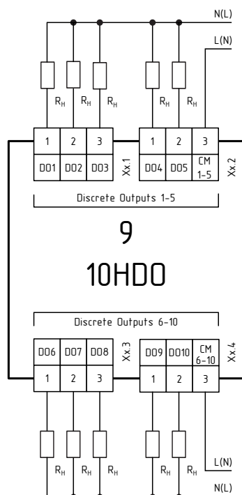
Рисунок 1.24 – Схема подключения модуля расширения MCU-9-10HDO
