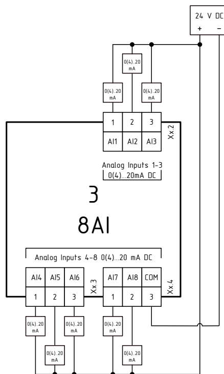
Рисунок 1.12 – Схема подключения модуля расширения MCU-3-8AI
