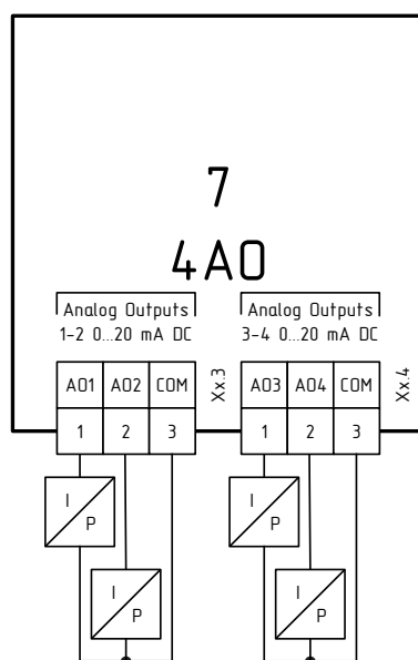
Рисунок 1.20 – Схема подключения модуля расширения MCU-7-4AO
