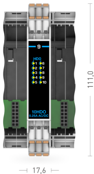
Рисунок 1.23 – Внешний вид модуля расширения MCU-9-10HDO
