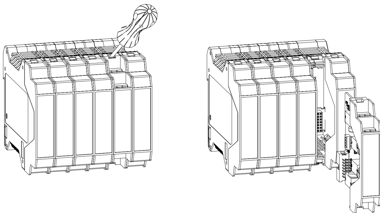
Рисунок 2.3 – Демонтаж модуля
